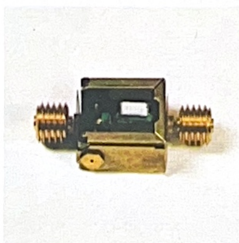
602 Elektromotor 12 V Flachbauweise mit 2 Schnecken
