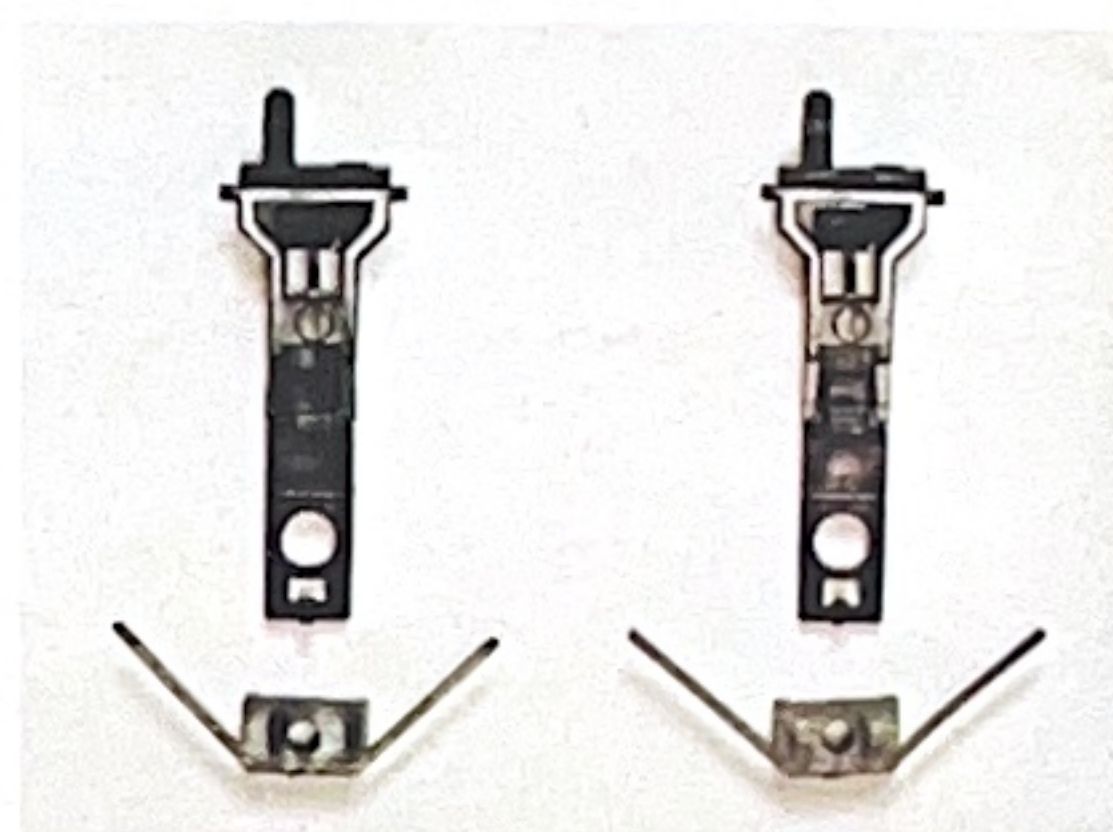
101 gogTram Kupplung einschließlich Rückstellfeder
